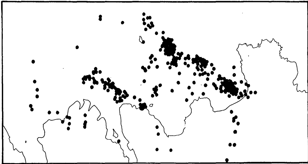
Mynd 6: Upptök jarðskjálfta fyrir Norðurlandi árin 1982-1985. Skjálftar á gosbeltinu og Tjörnes-þverbrotabeltinu (á hafsbotni) koma vel fram.
