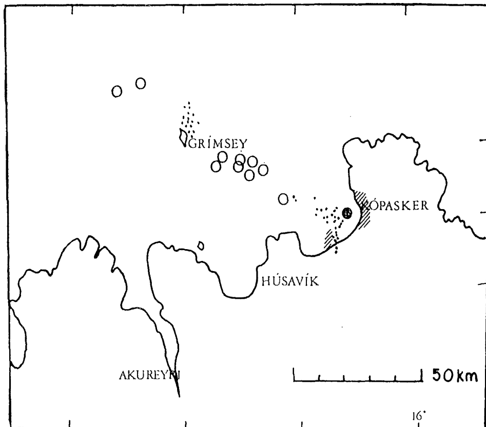
Mynd 7: Afstaða Kópaskersskjálftans, 13. janúar 1976 til Tjörnes-þverbrotabeltisins. Kópaskersskjálftinn er sýndur með svörtum punkti. Litlir punktar eru miðjur skjálfta sem fylgdu í kjölfarið í Öxarfirði og við Grímsey. Einnig eru sýndir á myndinni miðjur nokkurra annara jarðskjálfta sem orðið hafa á þverbrotabeltinu. Hreyfingarsvæði við Kópaskersskjálftann eru skástrikuð.
