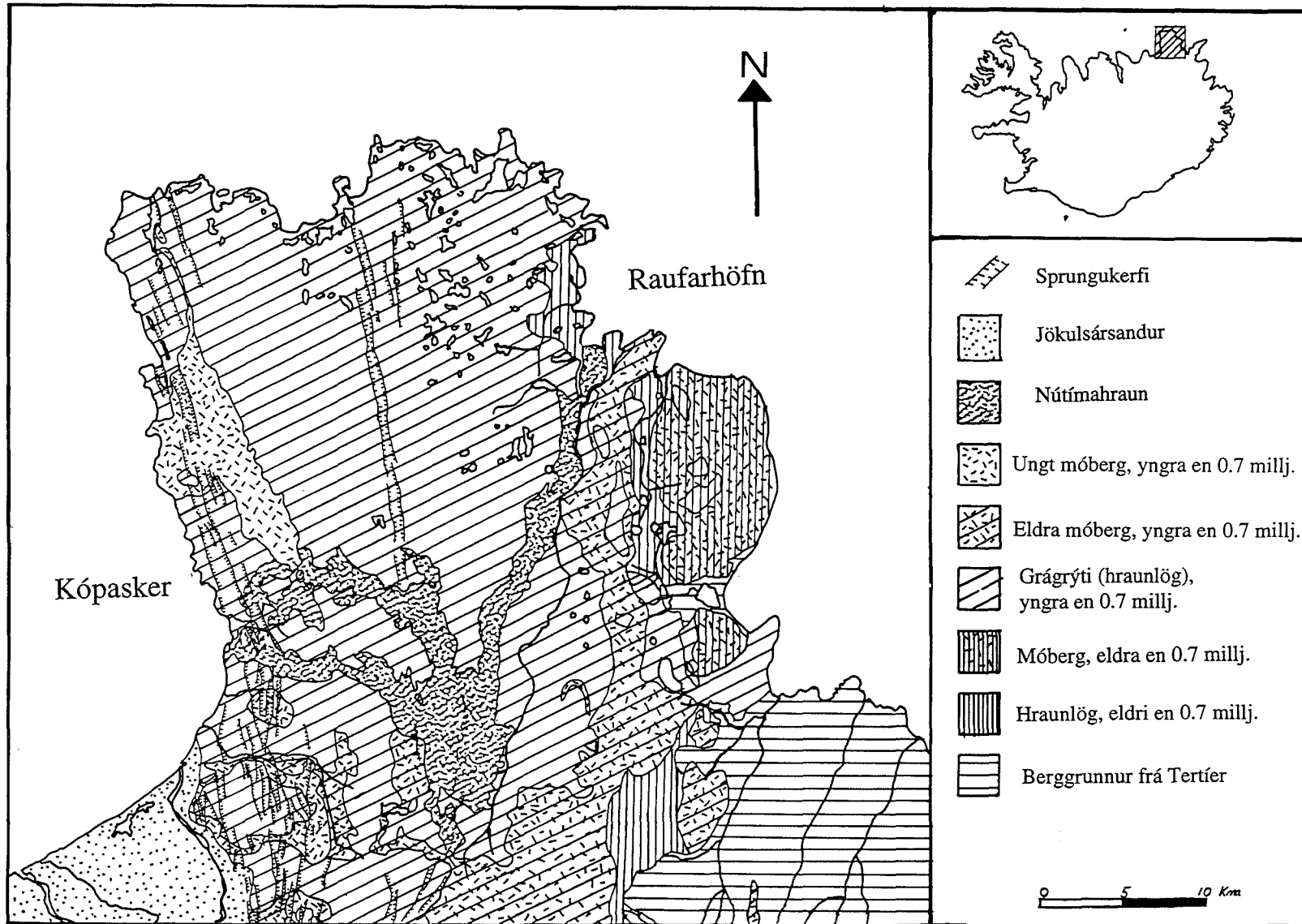
Mynd 3: Berggrunnskort af Melrakkasléttu.
