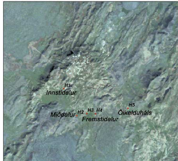
3. mynd. Jarðhitastaðir sem kannaðir voru á suðurhluta Hengilsvæðisins. Númer vísa til örnefna í texta. Gervitunglamynd frá Landmælingum Íslands.
