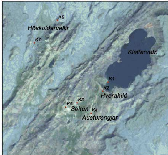
2. mynd. Jarðhitastaðir sem kannaðir voru á Krýsuvíkarsvæðinu. Númer vísa til örnefna í texta. Gervitunglamynd frá Landmælingum Íslands.
